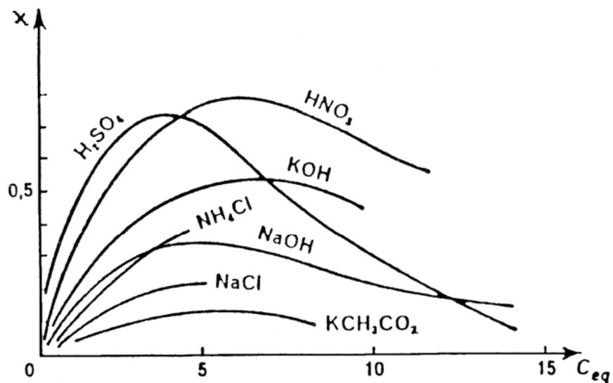
Fig. — Variazione della conduttività di alcune soluzioni acquose di elettroliti in funzione della concentrazione ( 18^{\circ}\text{C} ).
