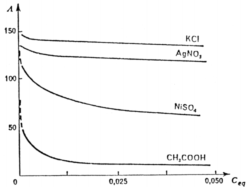
Fig. — Curve \lambda = \lambda(c_{eq}) per alcuni elettroliti ( 25^{\circ}\text{C} ).
