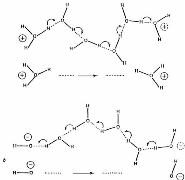
Fig. — Meccanismo di trasporto degli ioni H_3O^+ e OH^- per successivi trasferimenti di un protone da una molecola d'acqua ad un'altra.
